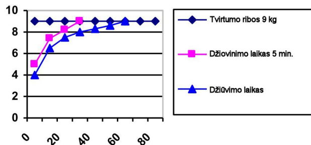
Galutinė SIMALFA® klijų sukibimo jėga
