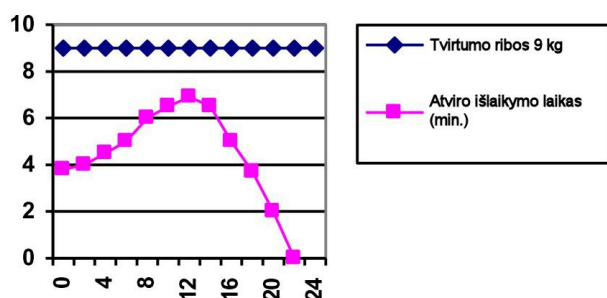
Pirminė SIMALFA® klijų sukibimo jėga
